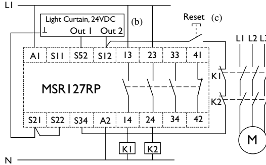
(d) Light Curtain, Manual Reset, Monitored Output
